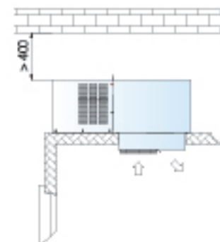
安装示意图 Installation sizes
